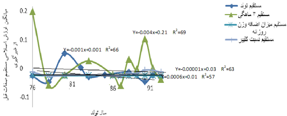
شکل ۲- روند ژنتیکی مستقیم صفات قبل از شیرگیری Figure 2. Direct genetic trend of trait before weaning
