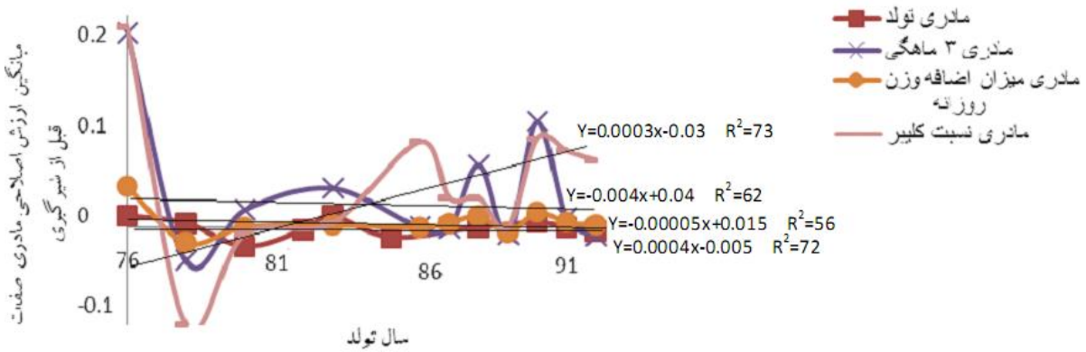
شکل ۳- روند ژنتیکی مادری صفات قبل از شیرگیری Figure 3. Maternal genetic trend of trait before weaning
