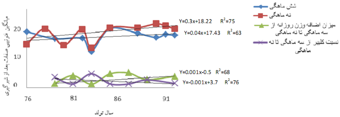
شکل ۴- روند فنوتیپی صفات بعد از شیرگیری Figure 4. Phenotypic trend of trait after weaning
