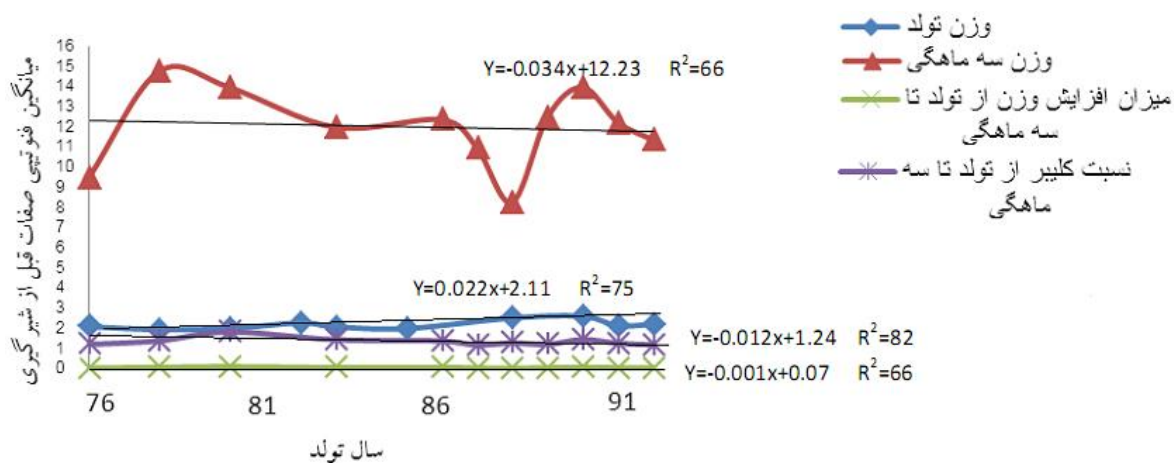
شکل ۱- روند فنوتیپی صفات قبل از شیرگیری Figure 1. Phenotypic trend of trait before Weaning
